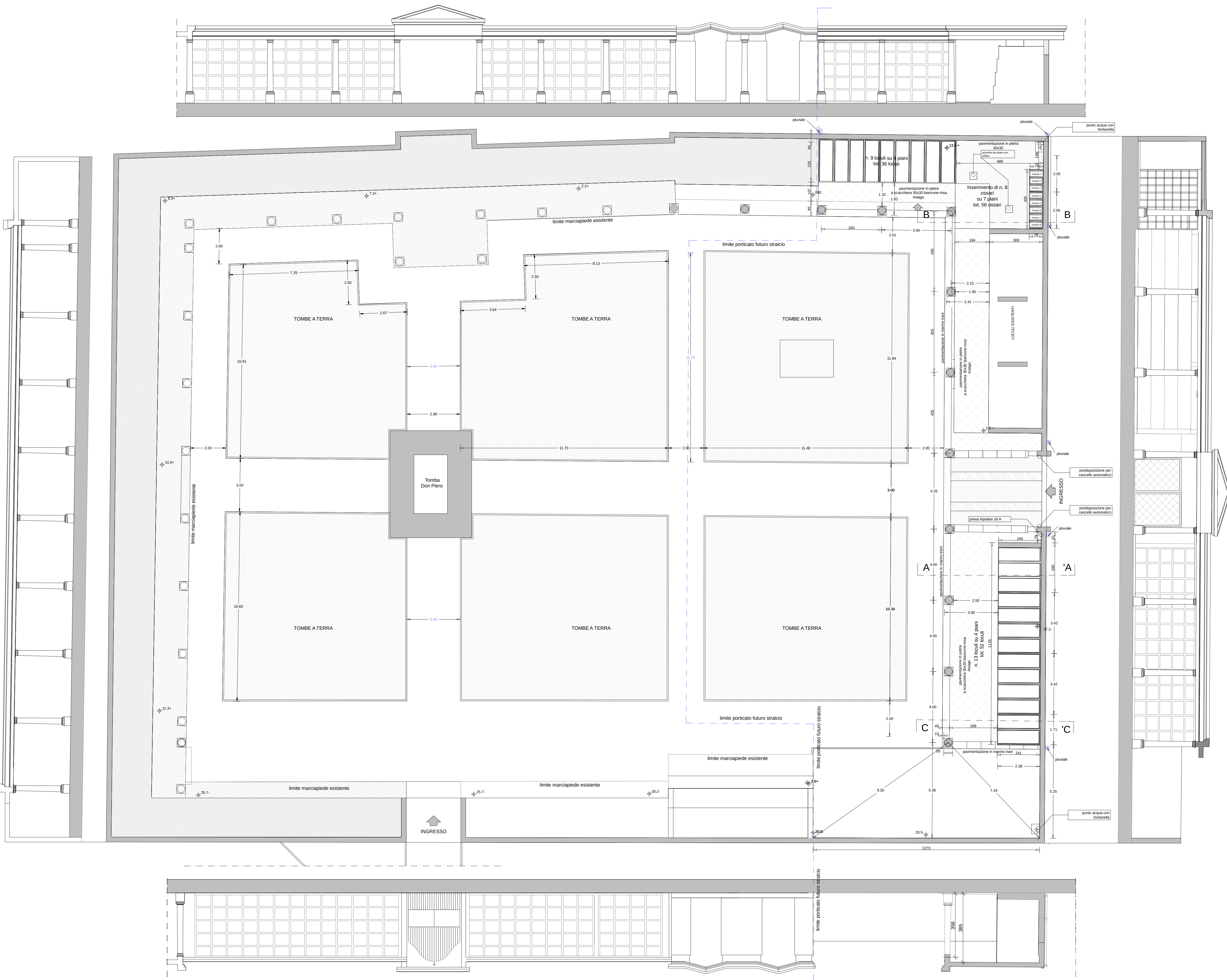
PIANTA E PROSPETTI scala 1:100
